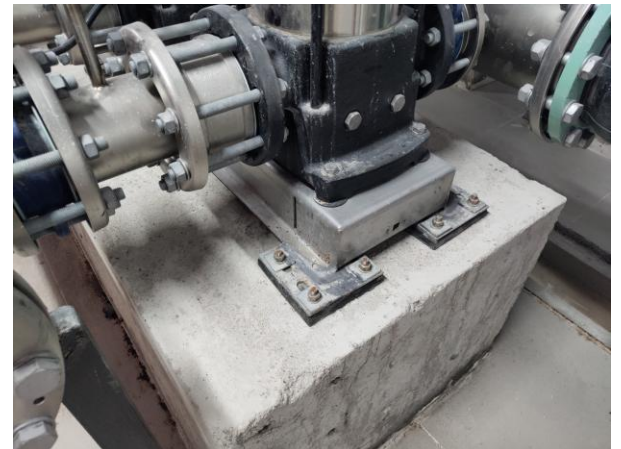
水泵减振垫
