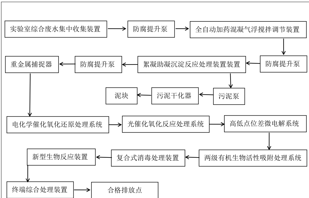
图 1 项目污水处理流程
