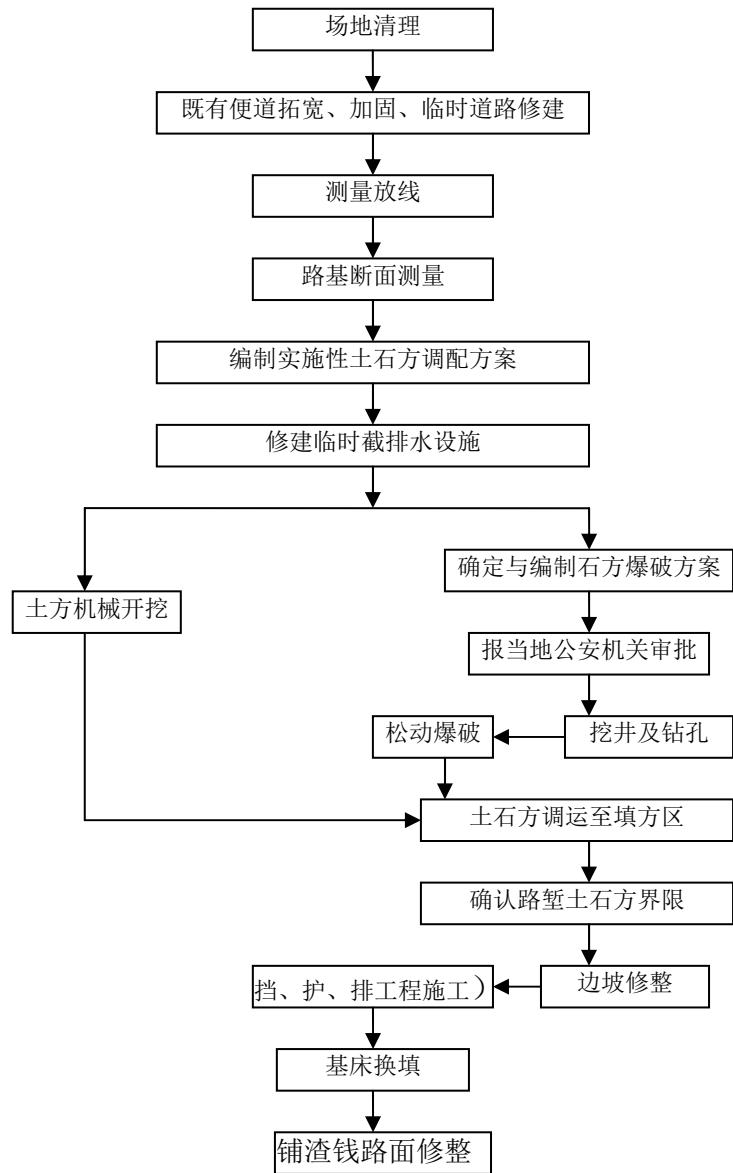
图 2.4-3 路堑开挖施工工艺流程
