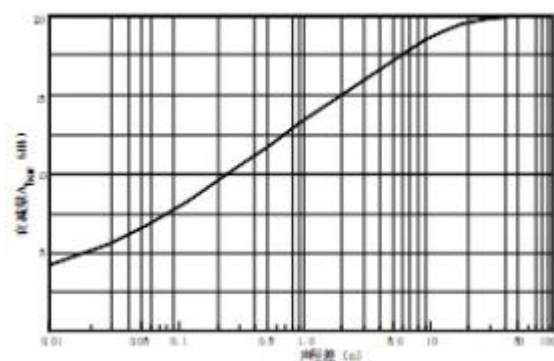
图4.1-1 声程差 \delta 与噪声衰减量 A_{\text{bar}}
