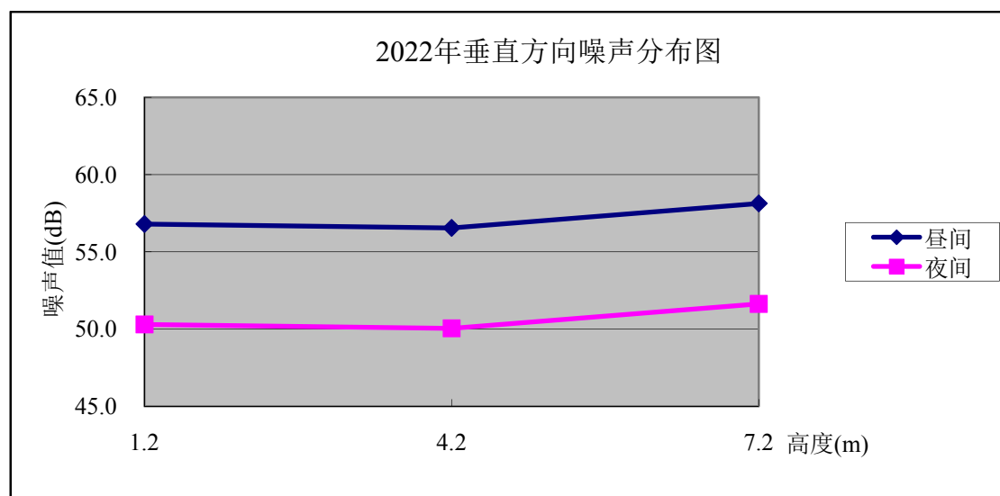
图 4.1-8 顶山前近期垂直方向噪声分布图
