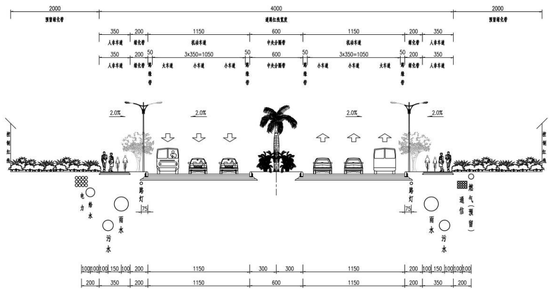
图2.3-2 道路标准横断面
