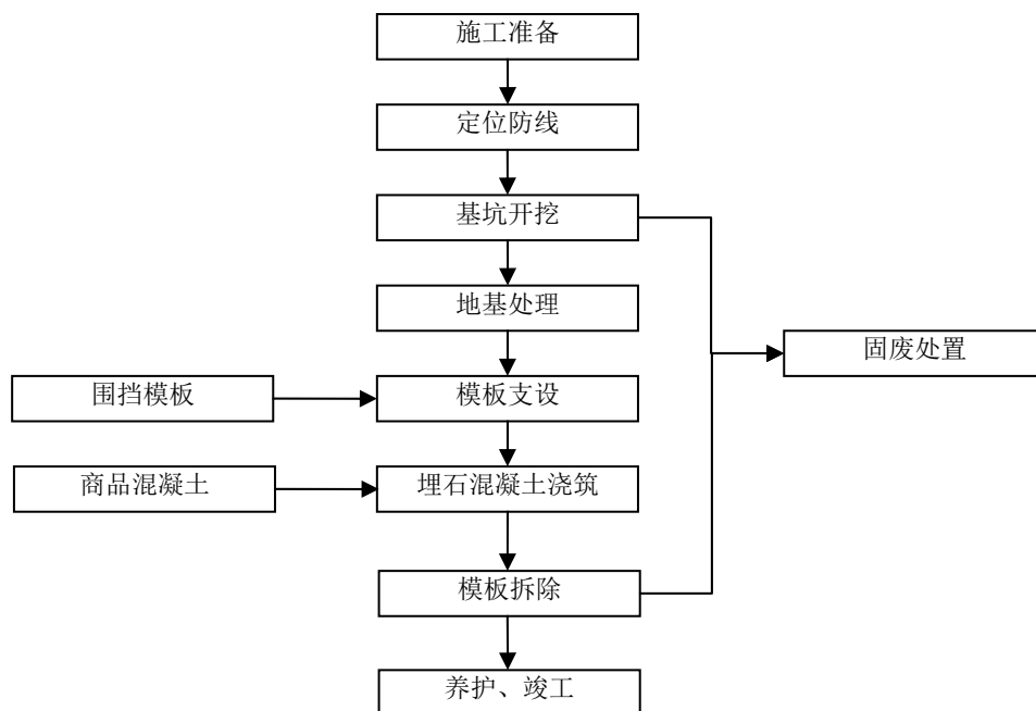
图 2.4-5 涵洞施工工艺流程
