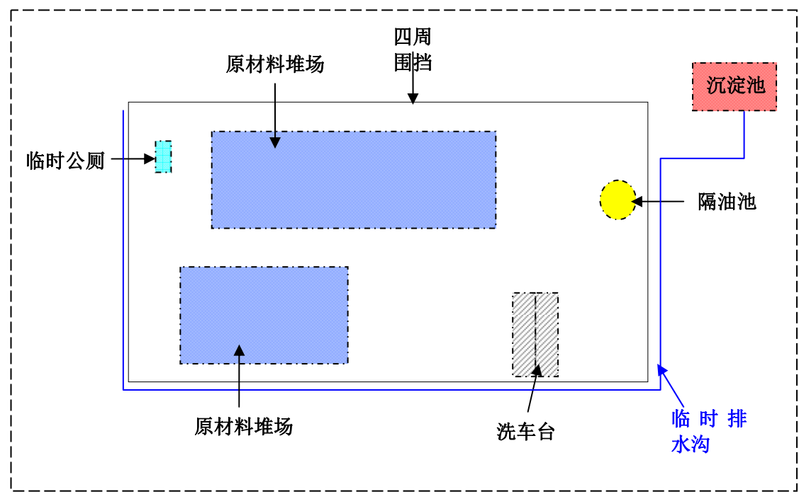
图2.4-1 施工场地内环保设施布置示意图
