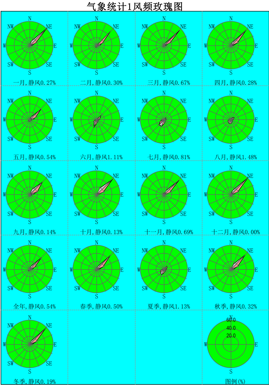
图 4.2-2 2019 全年风频率玫瑰图
