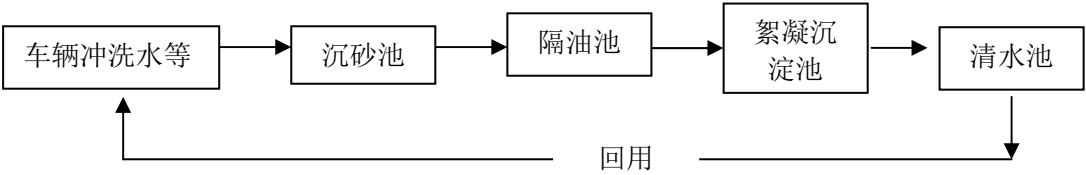
图 5.1-1 施工期废水处理工艺流程
