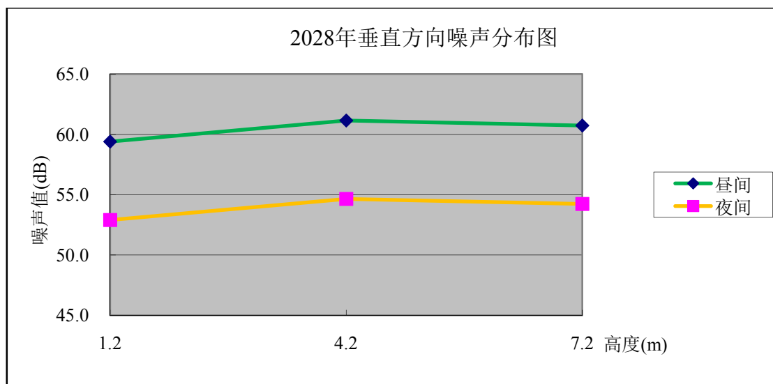
图 4.1-3 上山前中期垂直方向噪声分布图
