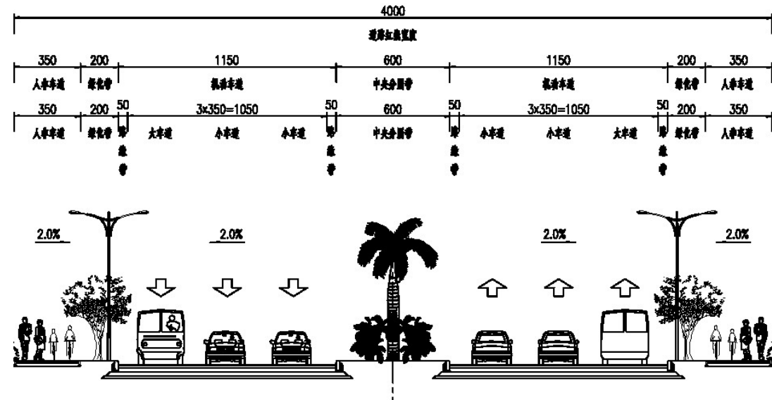
图2.3-1 道路标准横断面
