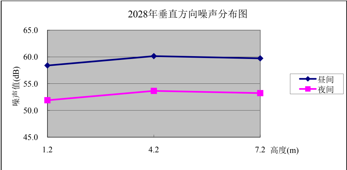
图 4.1-9 顶山前中期垂直方向噪声分布图
