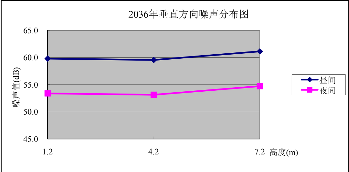
图 4.1-10 顶山前远期垂直方向噪声分布图
