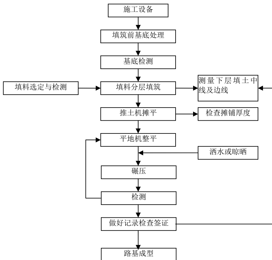
图 2.4-4 填筑路基施工工艺流程
