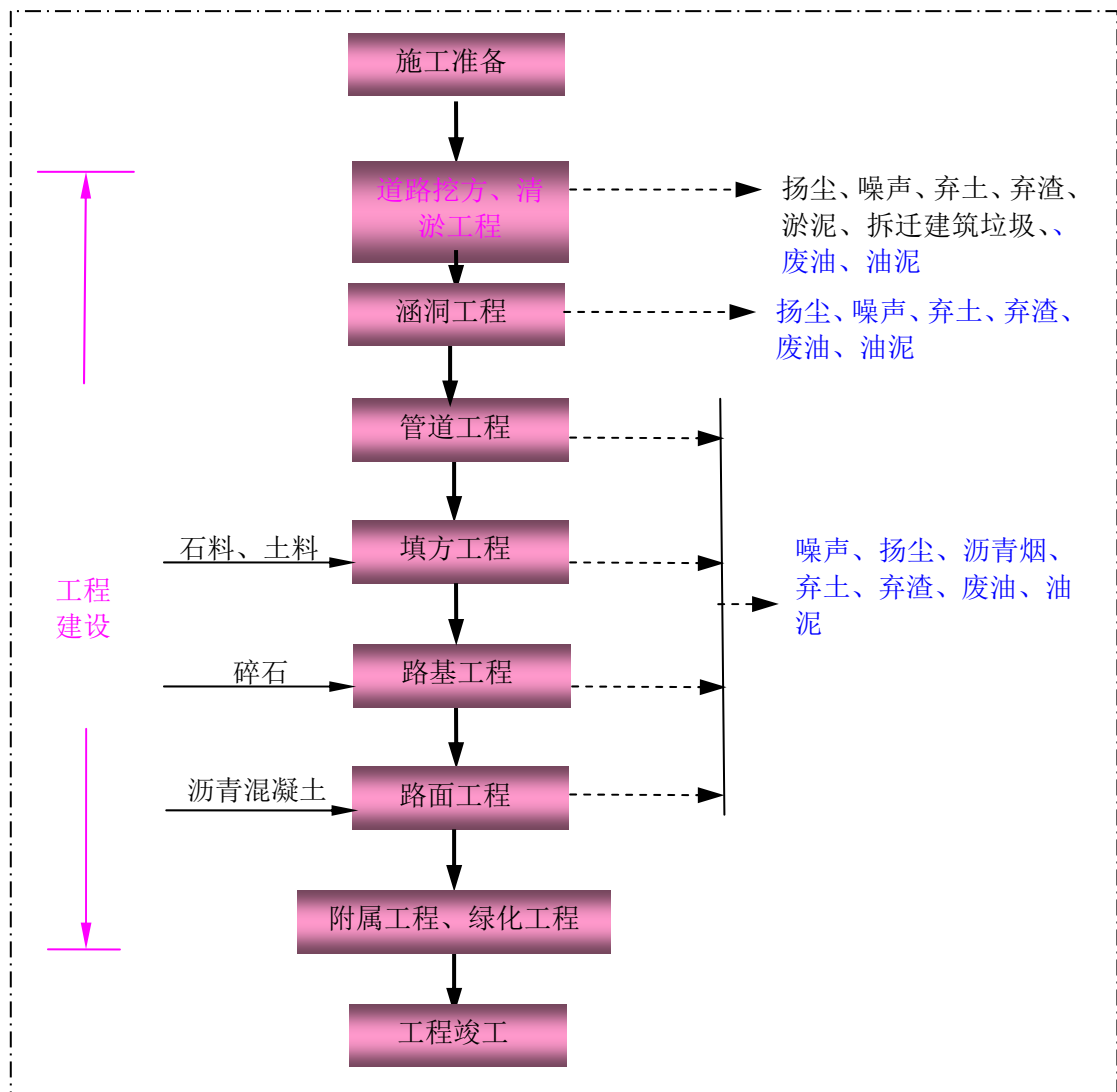
图2.4-2 工程施工工艺及产污环节图
