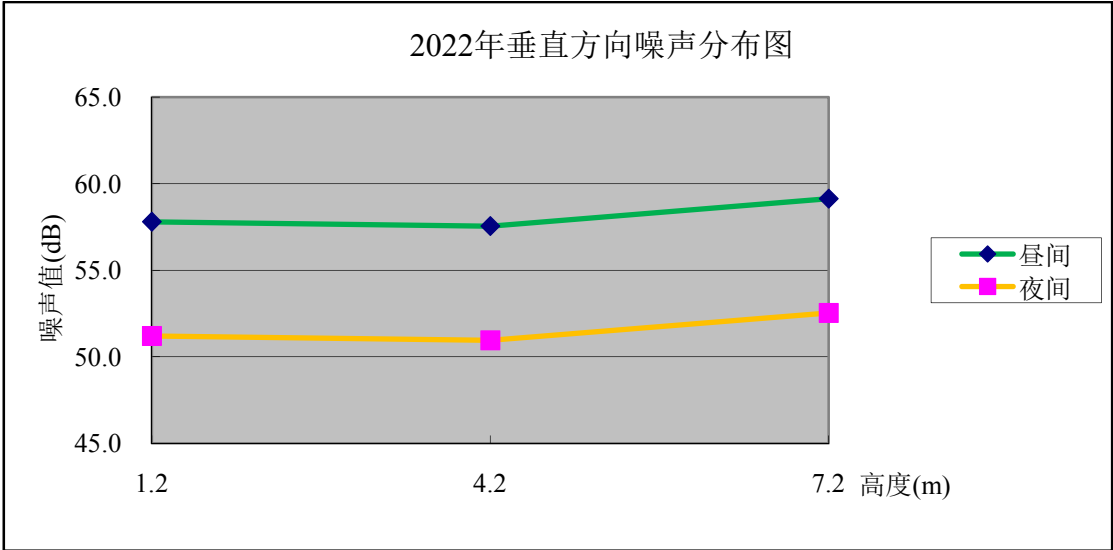
图 4.1-11 上山前近期垂直方向噪声分布图
