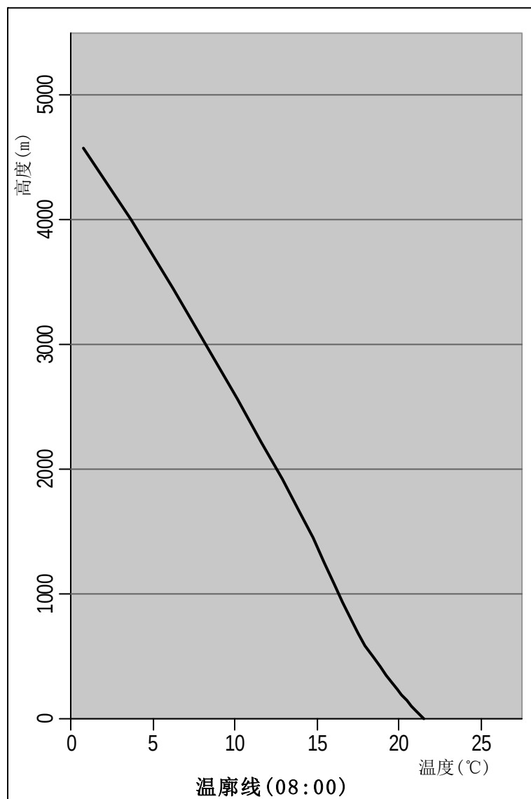
图 4.2-3 探空温廓线图
