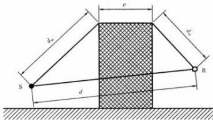
图4.1-2 双绕射预测
